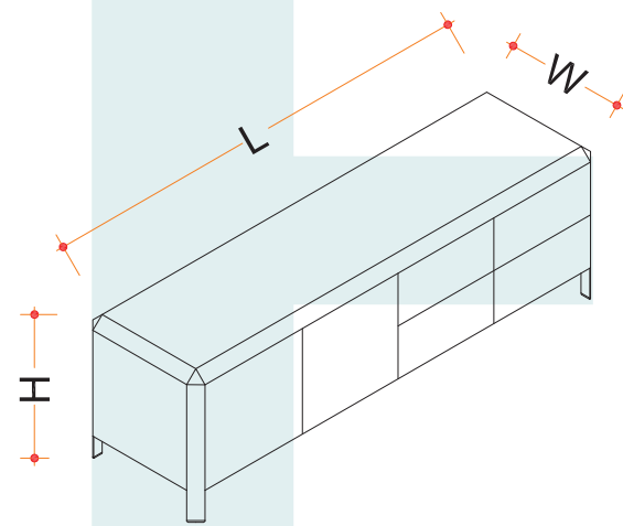
METİS YÖNETİCİ DOLABI WALL UNIT
