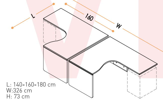
İKİLİ GRUP G MASALAR / DOUBLE GROUP TABLE - G TABLE
