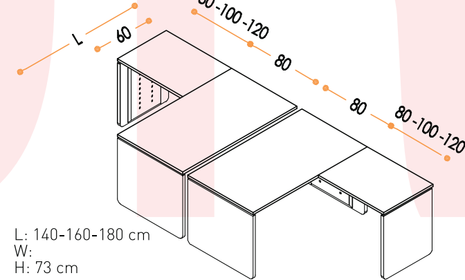
İKİLİ GRUP MASALAR / DOUBLE GROUP TABLE
