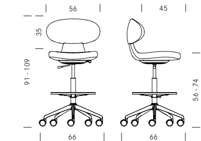
Simplex 3D çalışma koltuğu, yüksek Simplex 3D swivel chair, high
