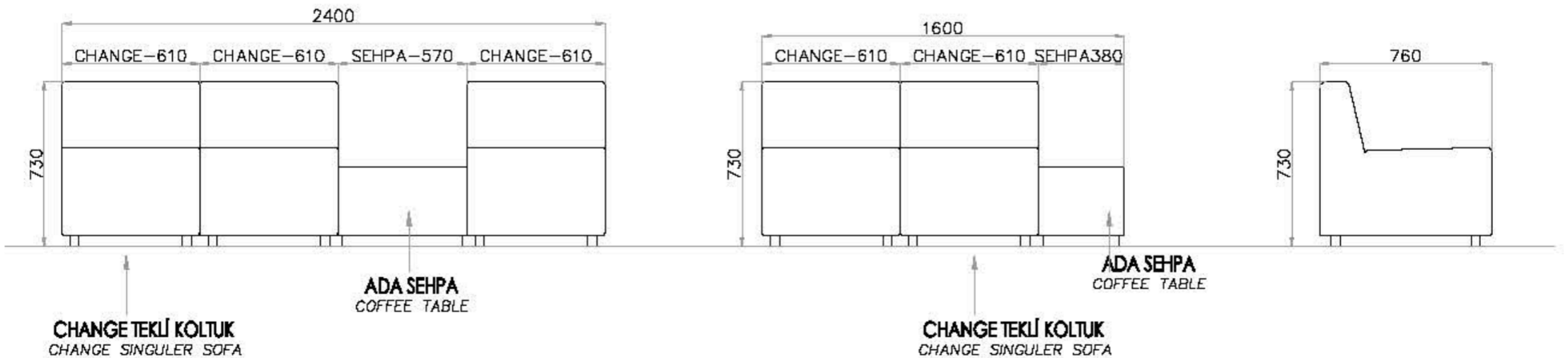
OTURMA MODÜLÜ ÖLÇÜLERİ SITTING SIDE SIZE
